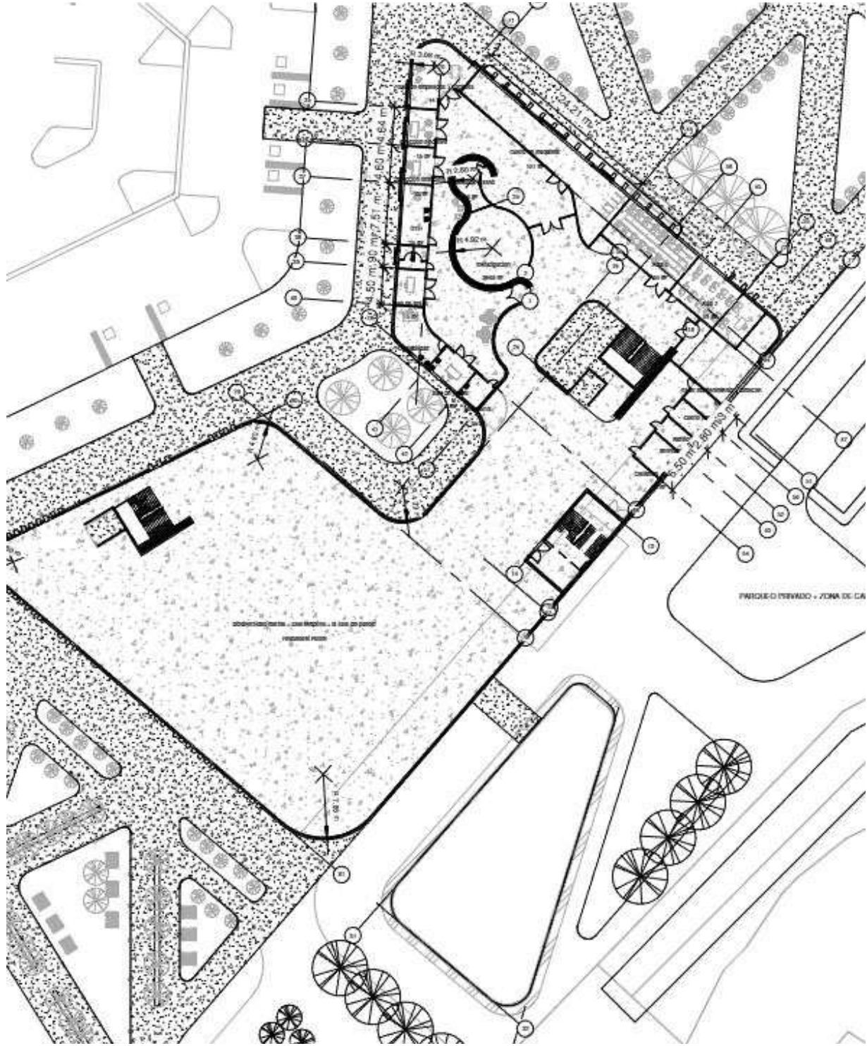
Planta arquitectónica Nivel 2 esc. 1:150
