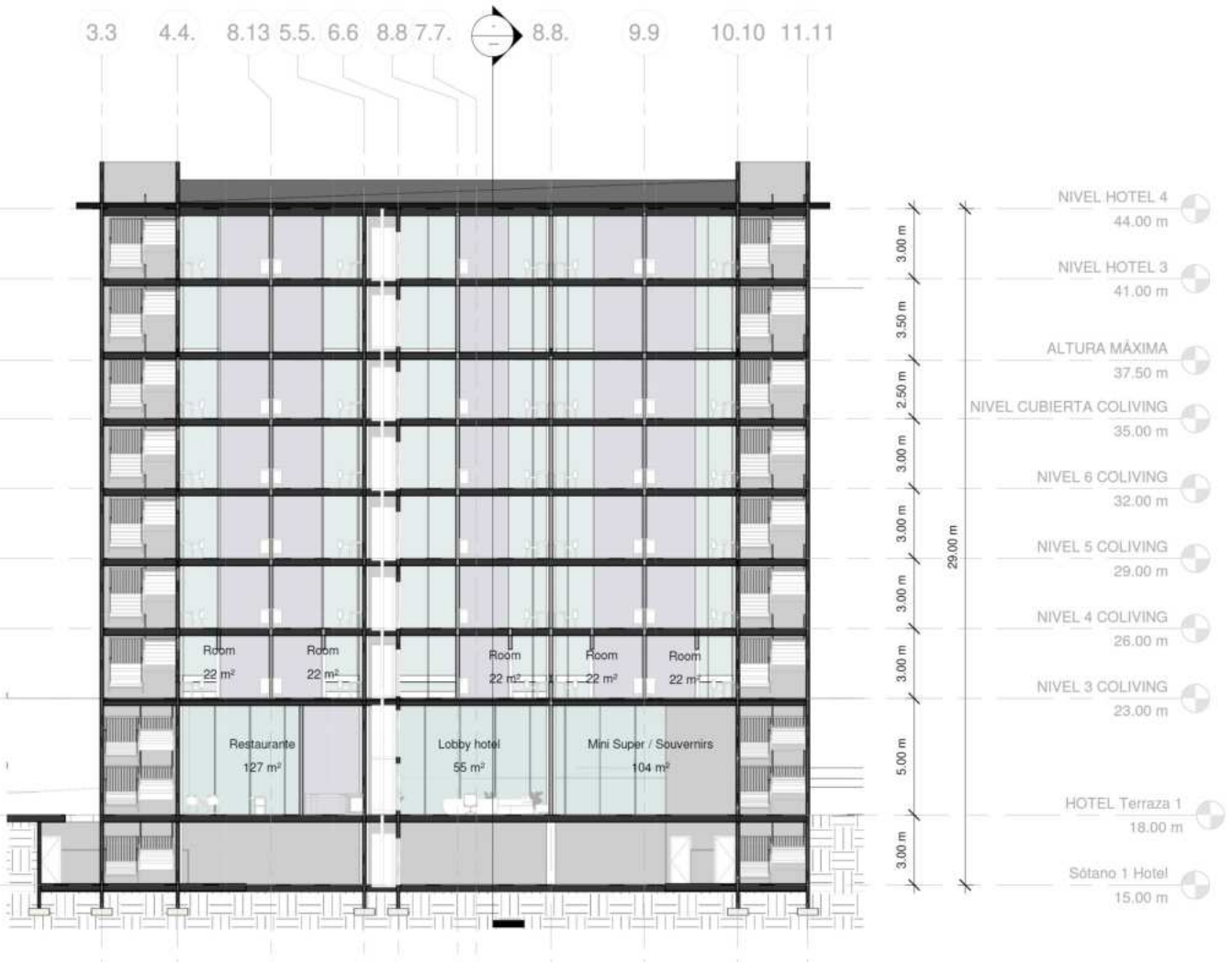
SECCIÓN LONGITUDINAL DEL HOTEL
