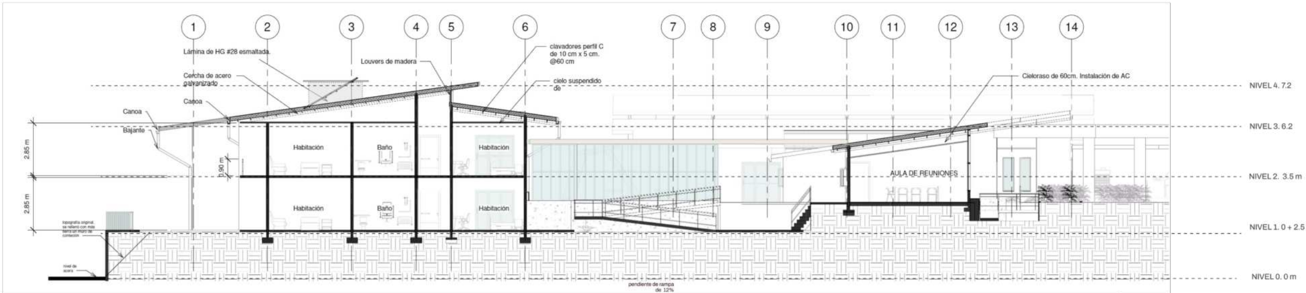
SECCIÓN B-B esc 1:100
