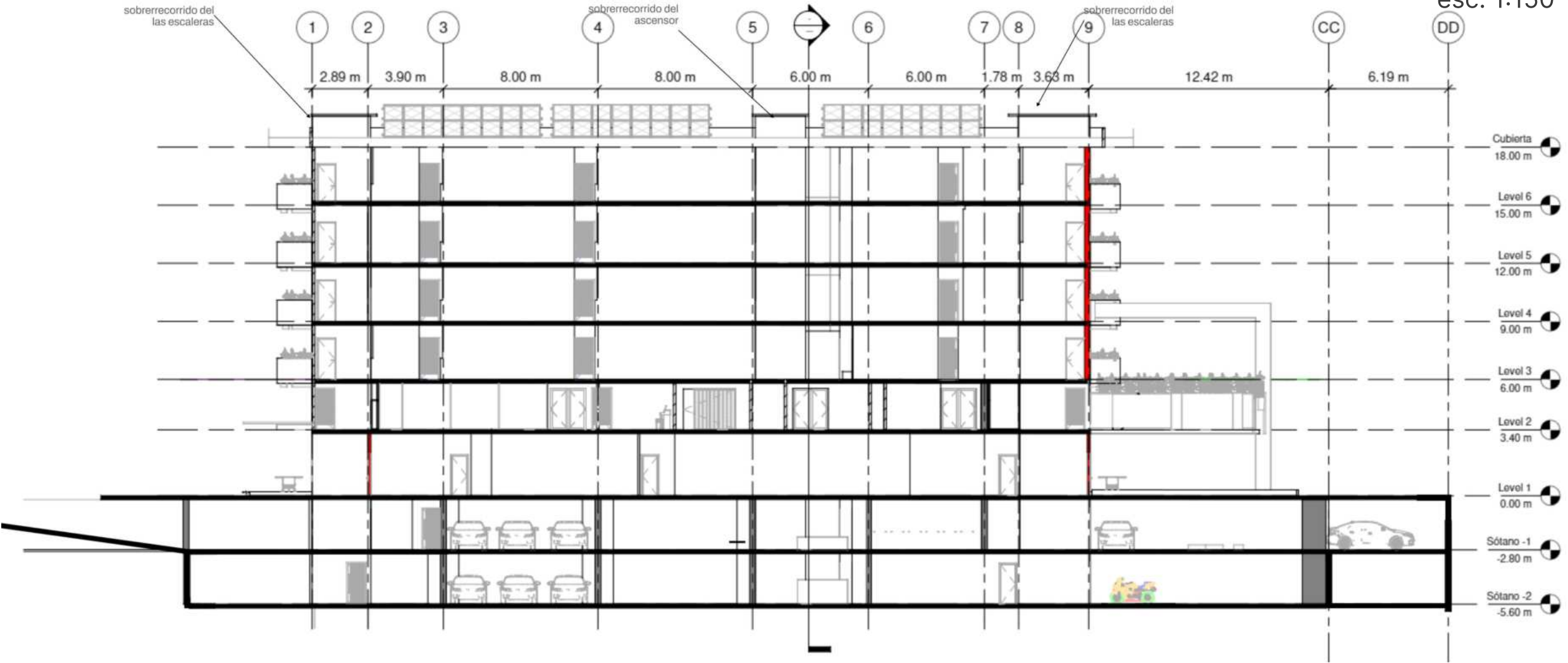
Sección transversal A-A esc. 1:150
