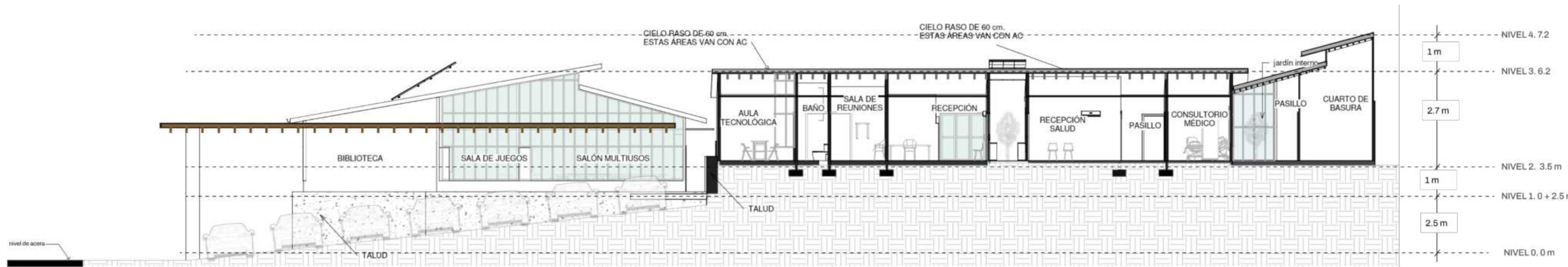
SECCIÓN A-A esc 1:100
