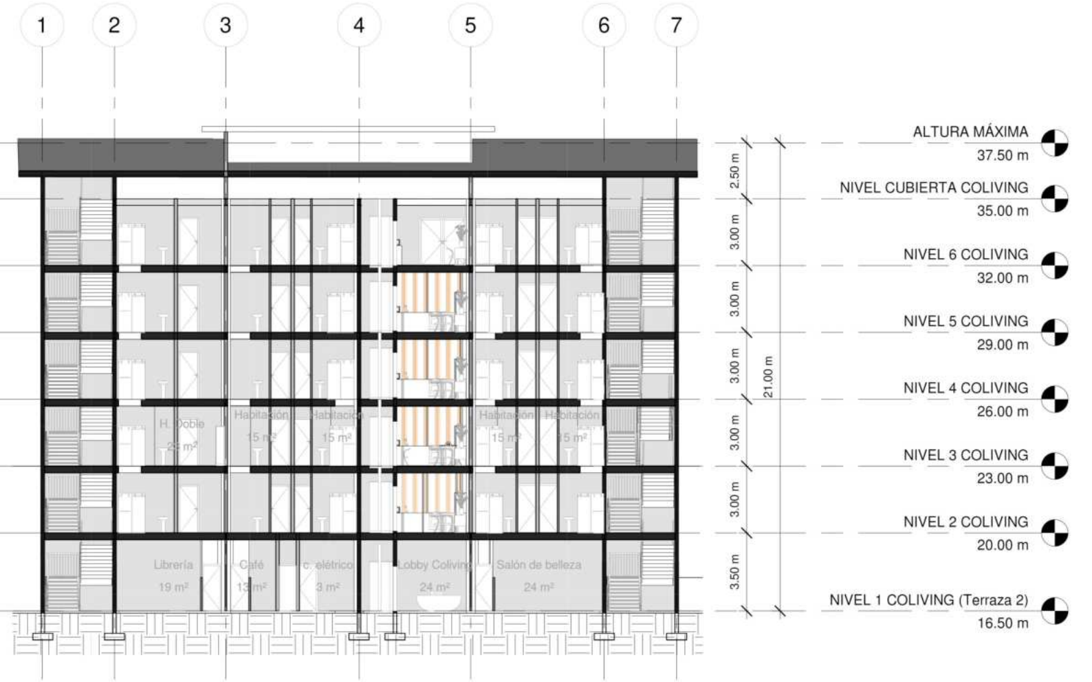
SECCIÓN LONGITUDINAL DEL COLIVING
