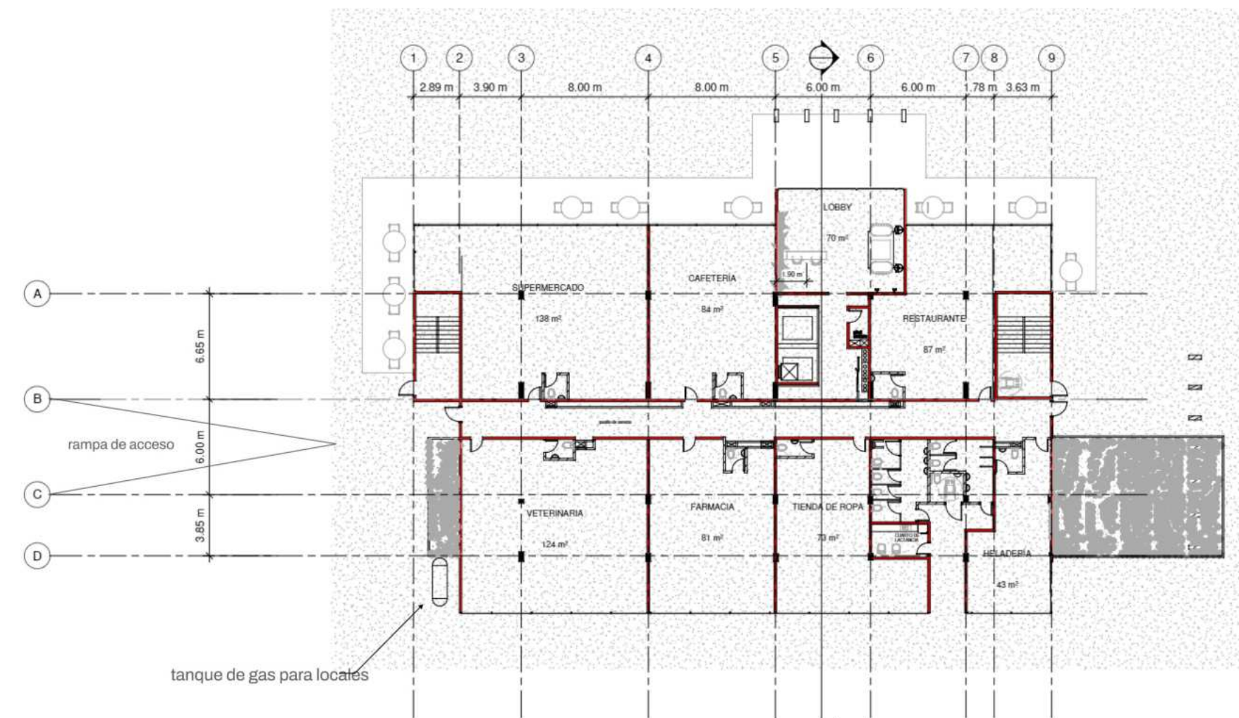
Planta 1. Comercial esc. 1:150
