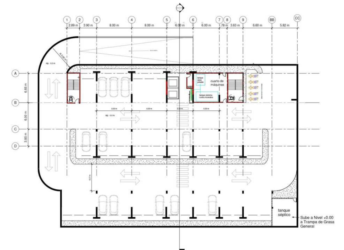
Sótano -2 esc. 1:150
