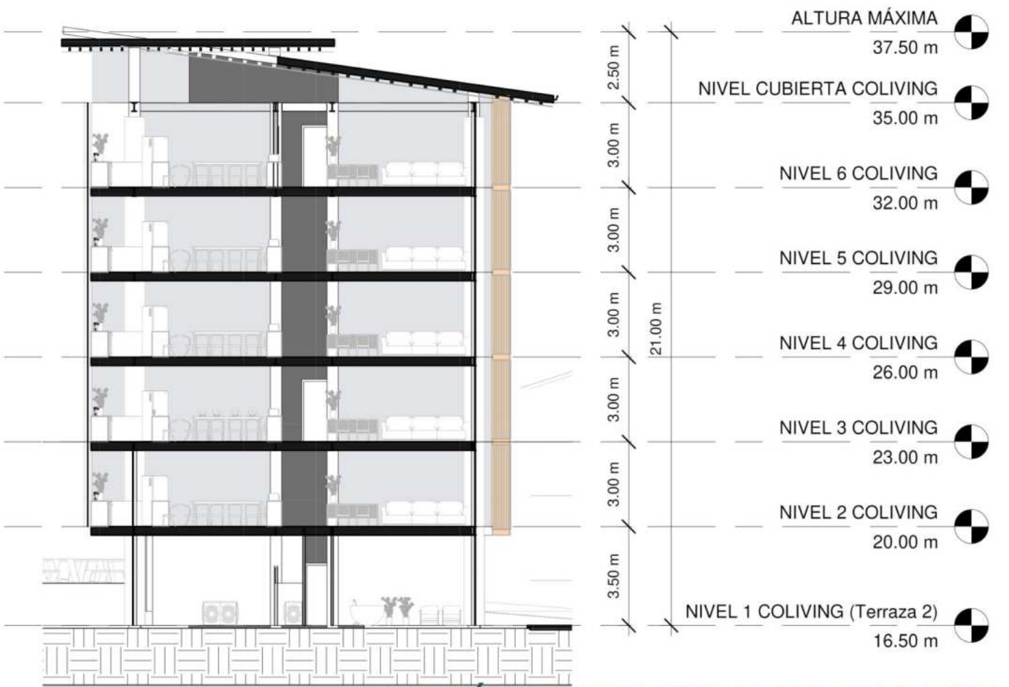
SECCIÓN TRANSVERSAL DEL COLIVING
